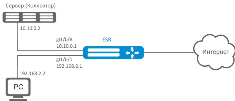
Рисунок 62 – Схема сети
