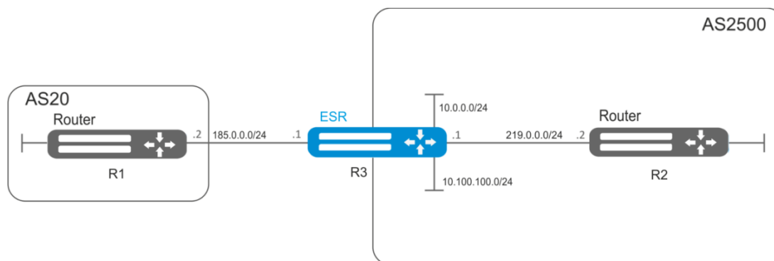
Рисунок 46 – Схема сети
