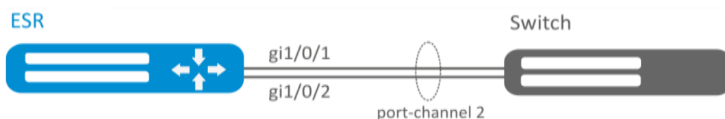
Рисунок 64 – Схема сети
