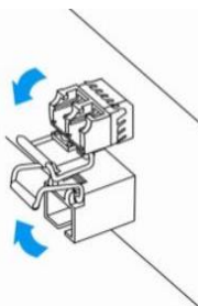
Рисунок 19 – Открытие защелки SFP-трансиверов
