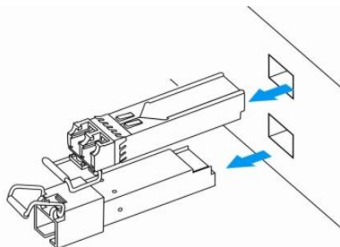
Рисунок 20 – Извлечение SFP-трансиверов
