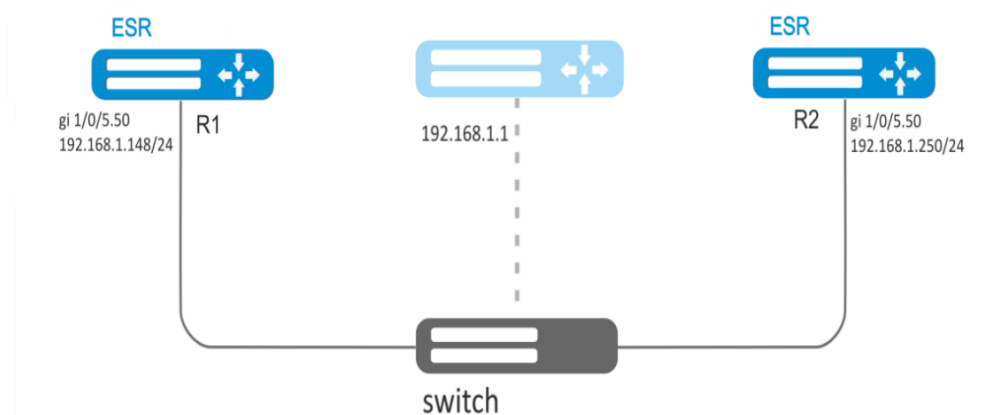
Рисунок 65 – Схема сети
