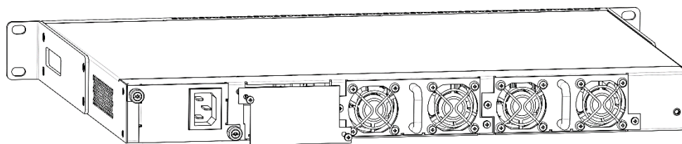
Рисунок 16 – Установка заглушки
