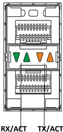
Рисунок 11 – Расположение индикаторов оптических интерфейсов
