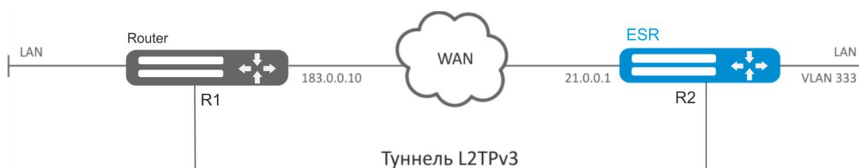
Рисунок 49 – Схема сети
