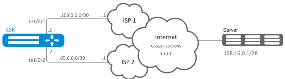
Рисунок 69 – Схема сети
