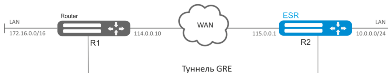
Рисунок 48 – Схема сети
