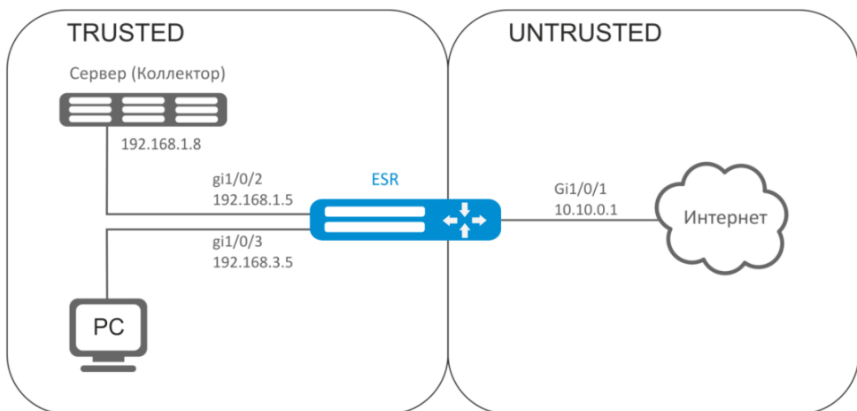
Рисунок 63 – Схема сети
