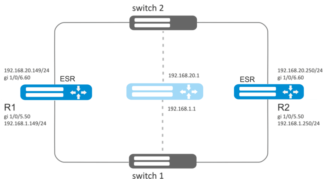
Рисунок 66 – Схема сети
