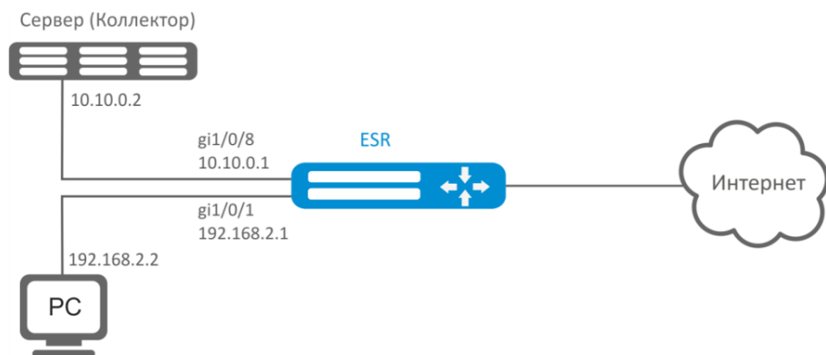
Рисунок 62 – Схема сети
