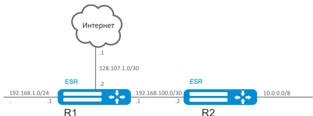
Рисунок 34 – Схема сети
