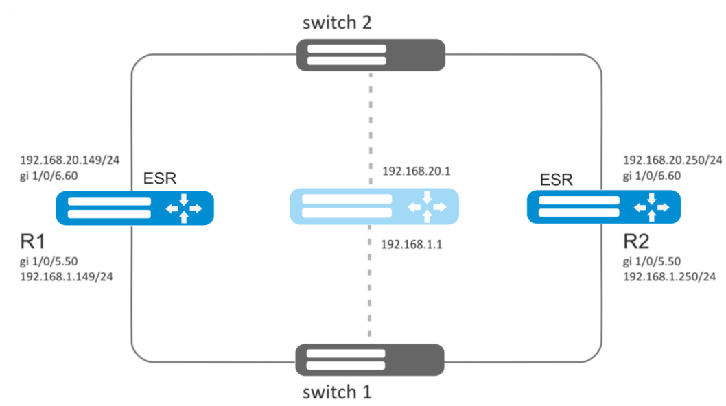
Рисунок 10.32 – Схема сети
