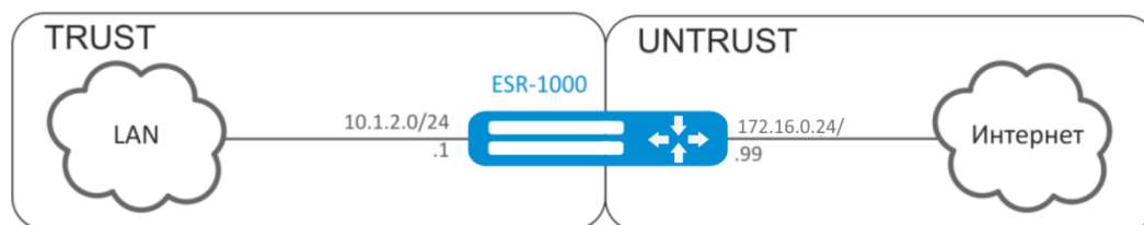
Рисунок 10.5 – Схема сети
