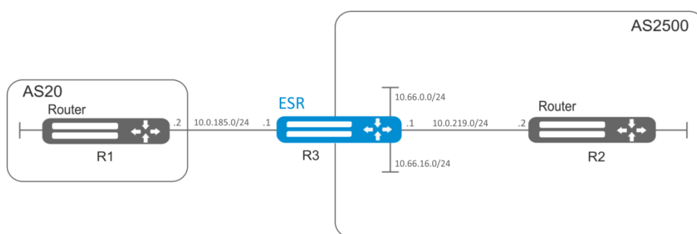
Рисунок 10.19 – Схема сети
