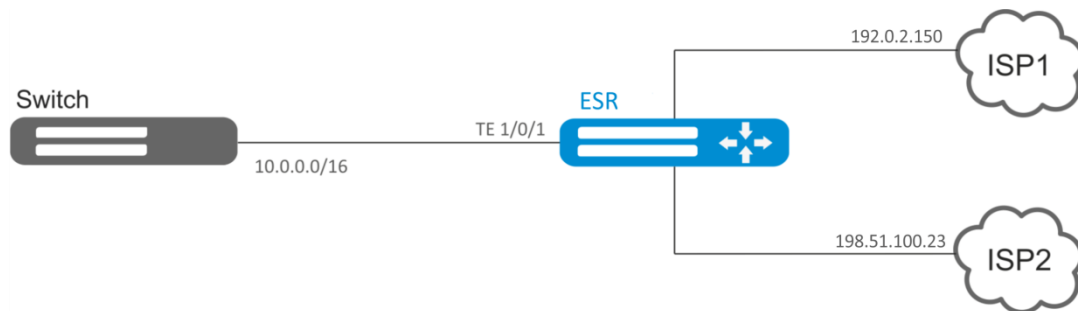
Рисунок 10.21 – Схема сети
