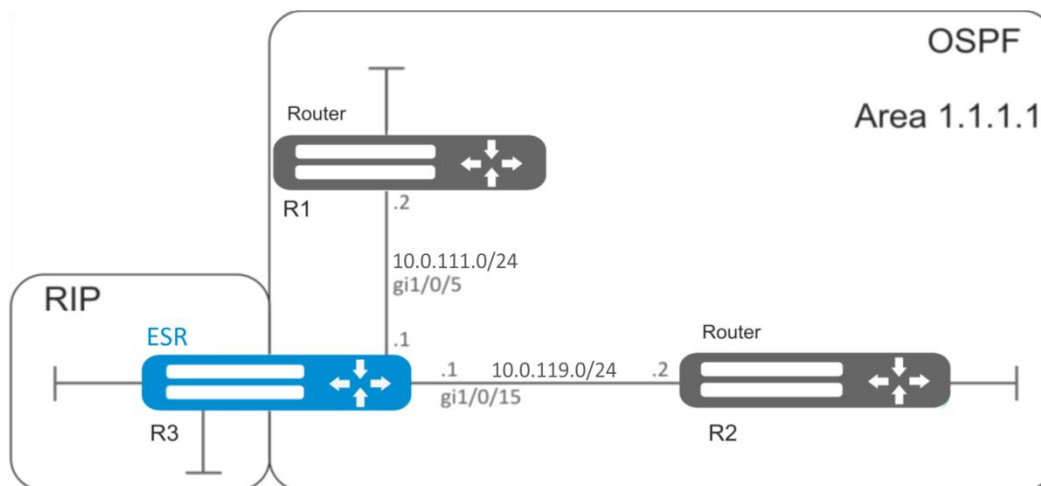
Рисунок 10.14 – Схема сети
