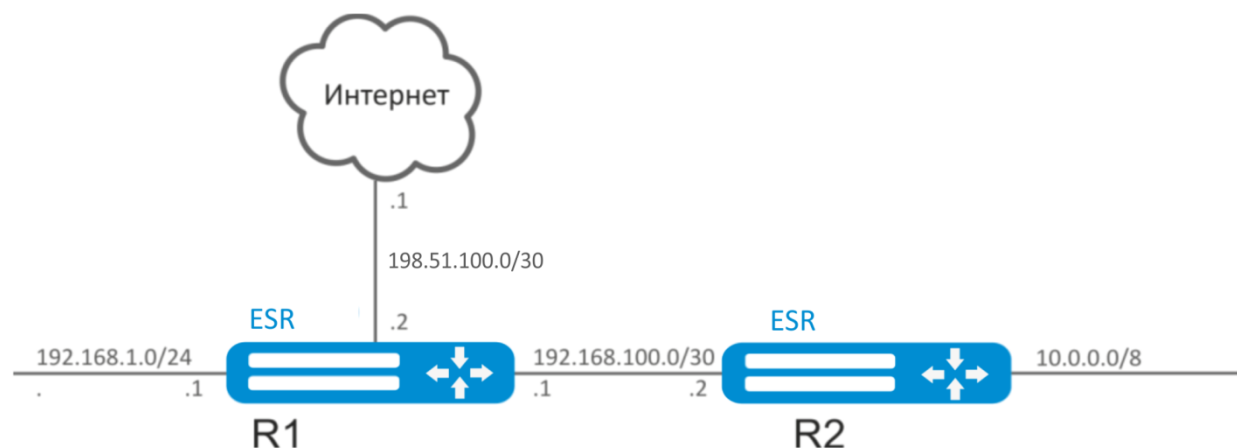
Рисунок 10.8 – Схема сети
