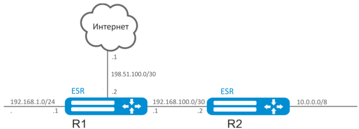
Рисунок 10.8 – Схема сети
