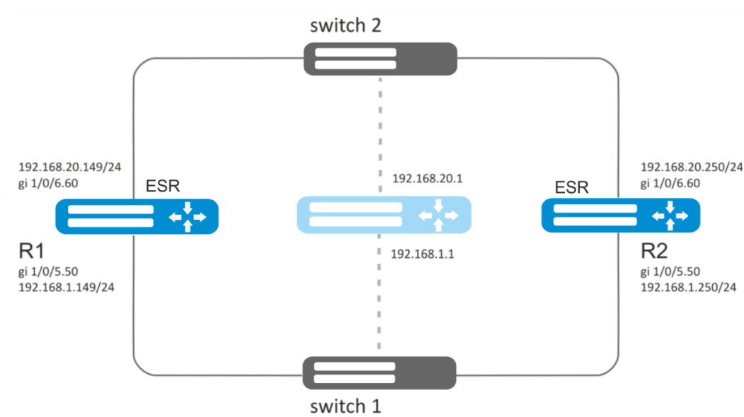
Рисунок 10.32 – Схема сети
