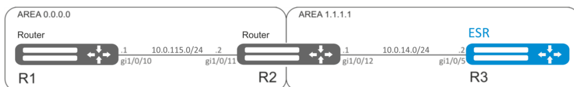
Рисунок 10.16 – Схема сети
