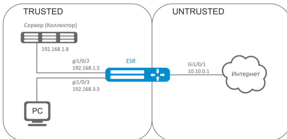
Рисунок 10.29 – Схема сети
