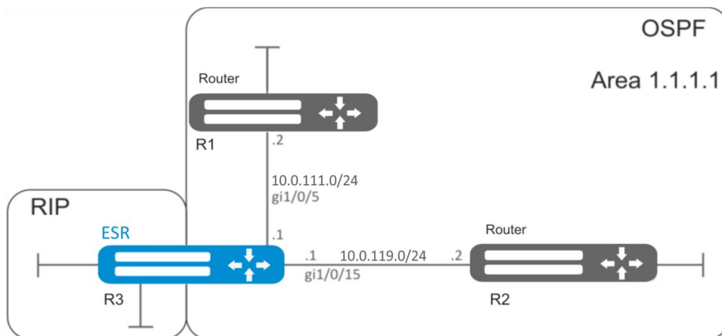
Рисунок 10.14 – Схема сети
