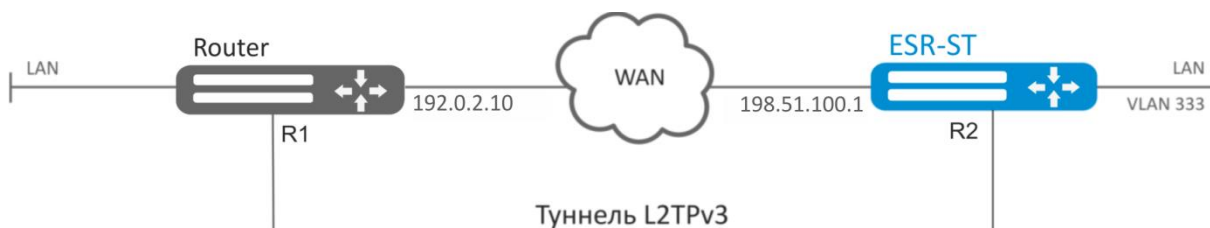
Рисунок 10.23 – Схема сети
