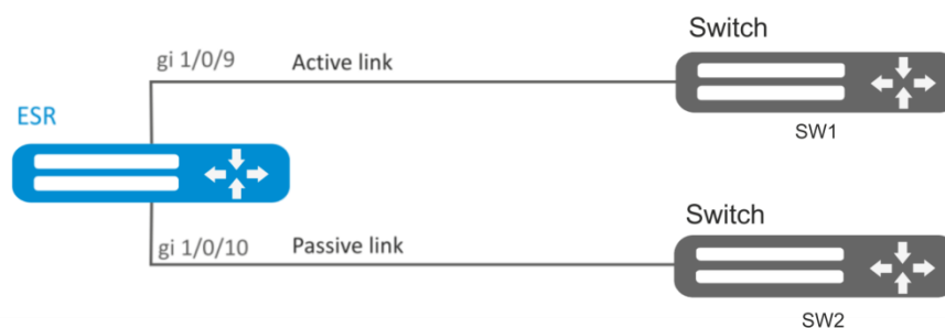
Рисунок 10.24 – Схема сети
