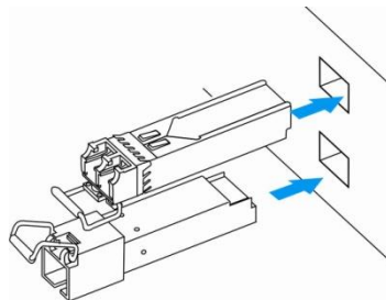
Рисунок 6.5 – Установка SFP-трансиверов
