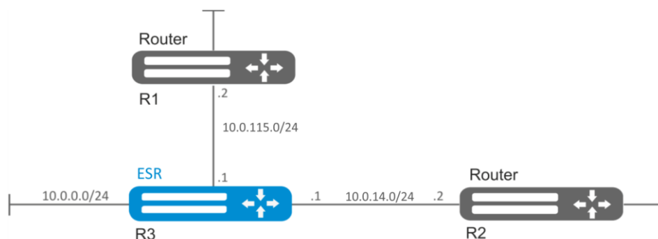
Рисунок 10.12 – Схема сети
