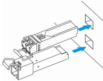
Рисунок 6.5 – Установка SFP-трансиверов
