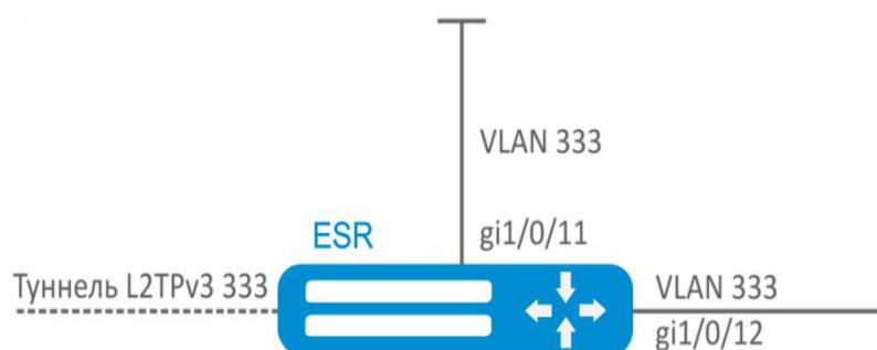
Рисунок 10.10 – Схема сети
