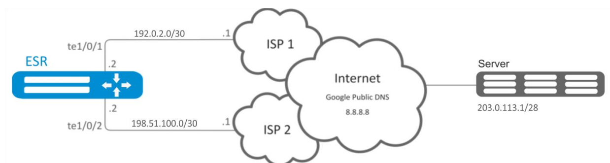
Рисунок 10.33 – Схема сети
