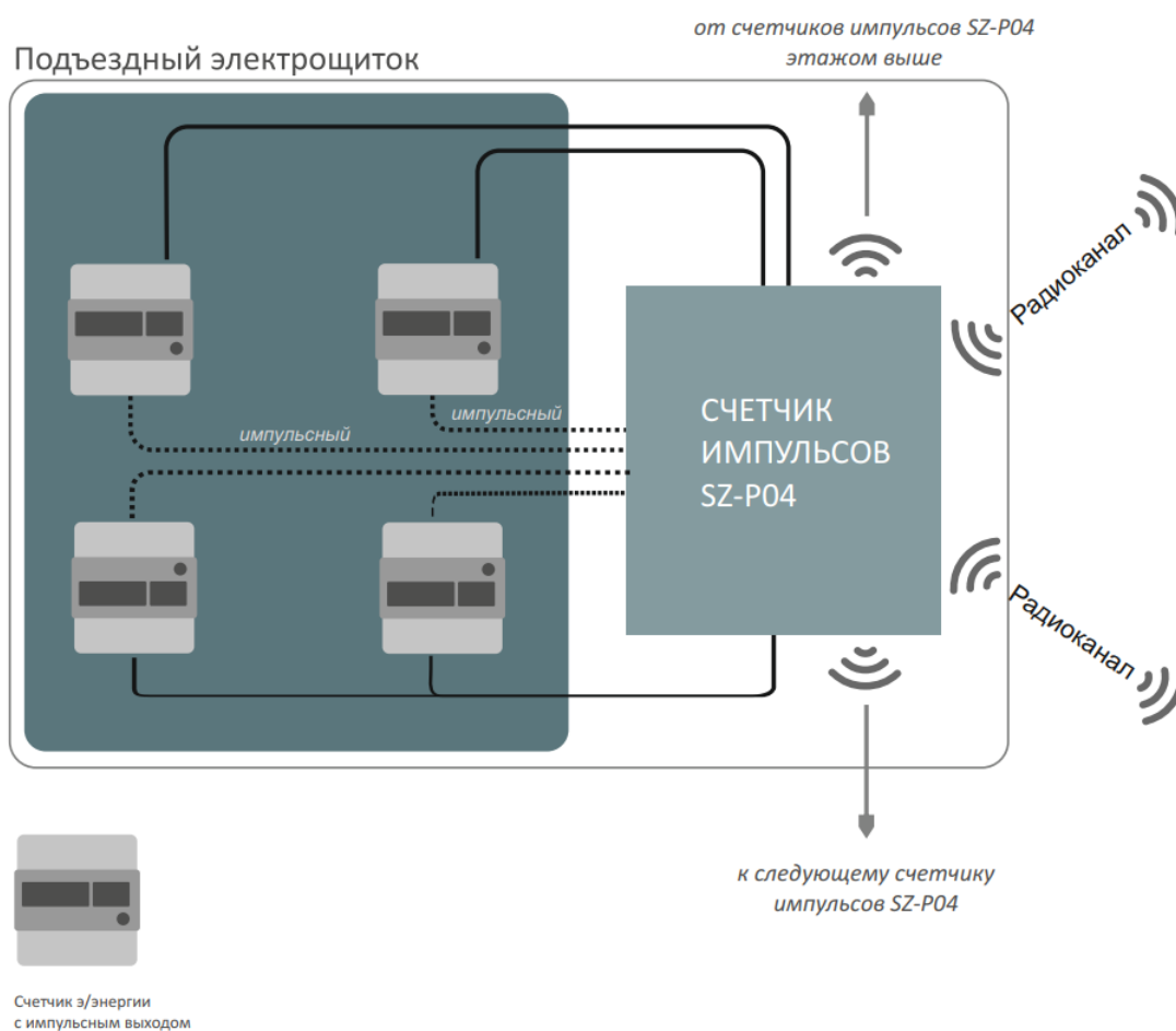
Рисунок 2 - Схема применения
