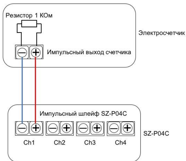
Рисунок 4 - Схема подключения
