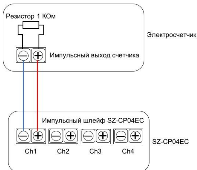
Рисунок 6 — Схема подключения
