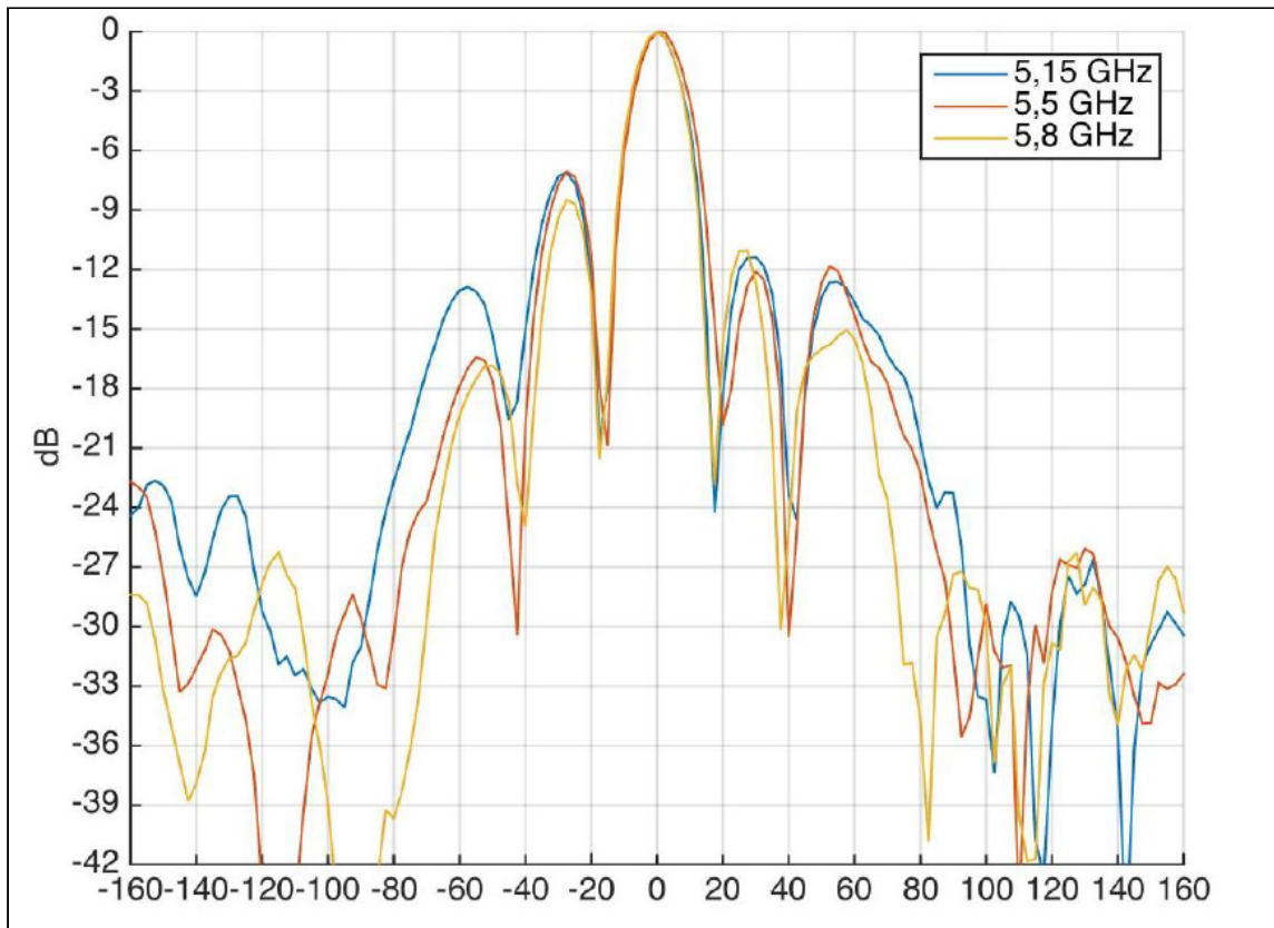
Диаграмма направленности антенны горизонтальной поляризации в E-плоскости:
