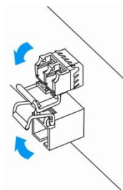
Рисунок 47 — Открытие защелки SFP-трансиверов
