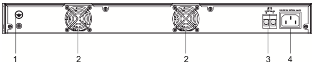
Рисунок 31 — Задняя панель MES2348B
