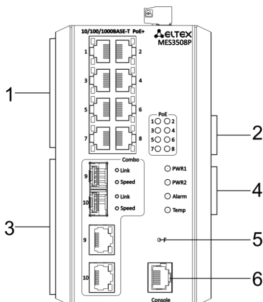
Рисунок 20 — Передняя панель MES3508P
