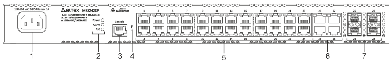
Рисунок 14 — Передняя панель MES2428P AC
