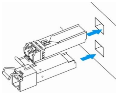
Рисунок 36 – Установка SFP-трансиверов
