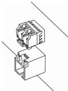
Рисунок 37 – Установленные SFP-трансиверы
