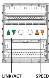
Рисунок 37 — Внешний вид разъема с QSPF+-трансиверами
