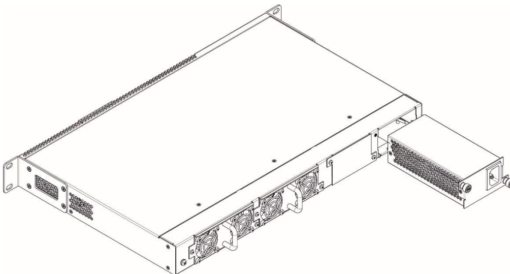
Рисунок 43 — Установка модулей питания
