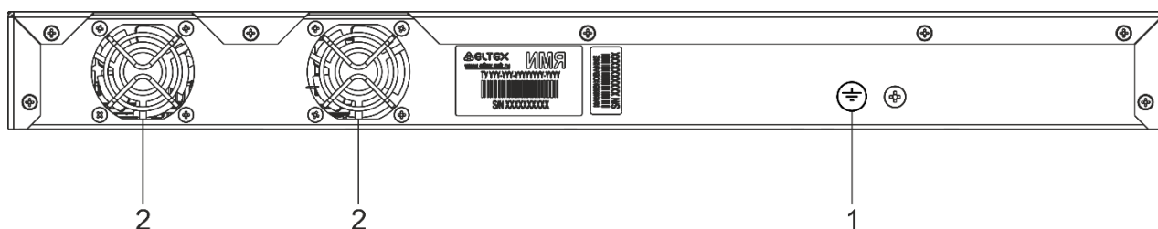
Рисунок 29 — Задняя панель MES2324P ACW
