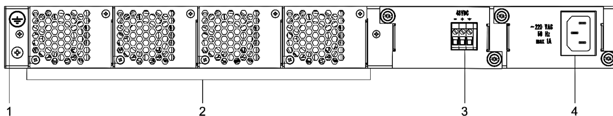
Рисунок 23 — Задняя панель MES3324F, MES3348F, MES3324
