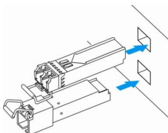
Рисунок 18 – Установка SFP-трансиверов
