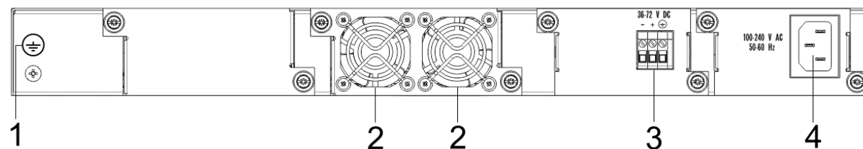
Рисунок 6 – Задняя панель MES5316A
