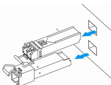
Рисунок 21 – Извлечение SFP-трансиверов
