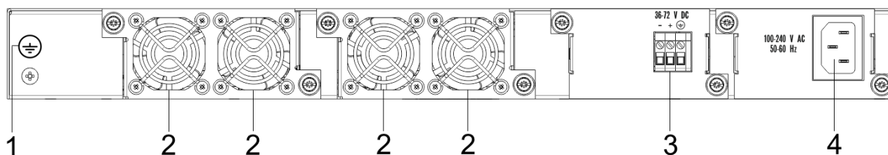
Рисунок 5 – Задняя панель MES5312, MES5324A, MES5332A
