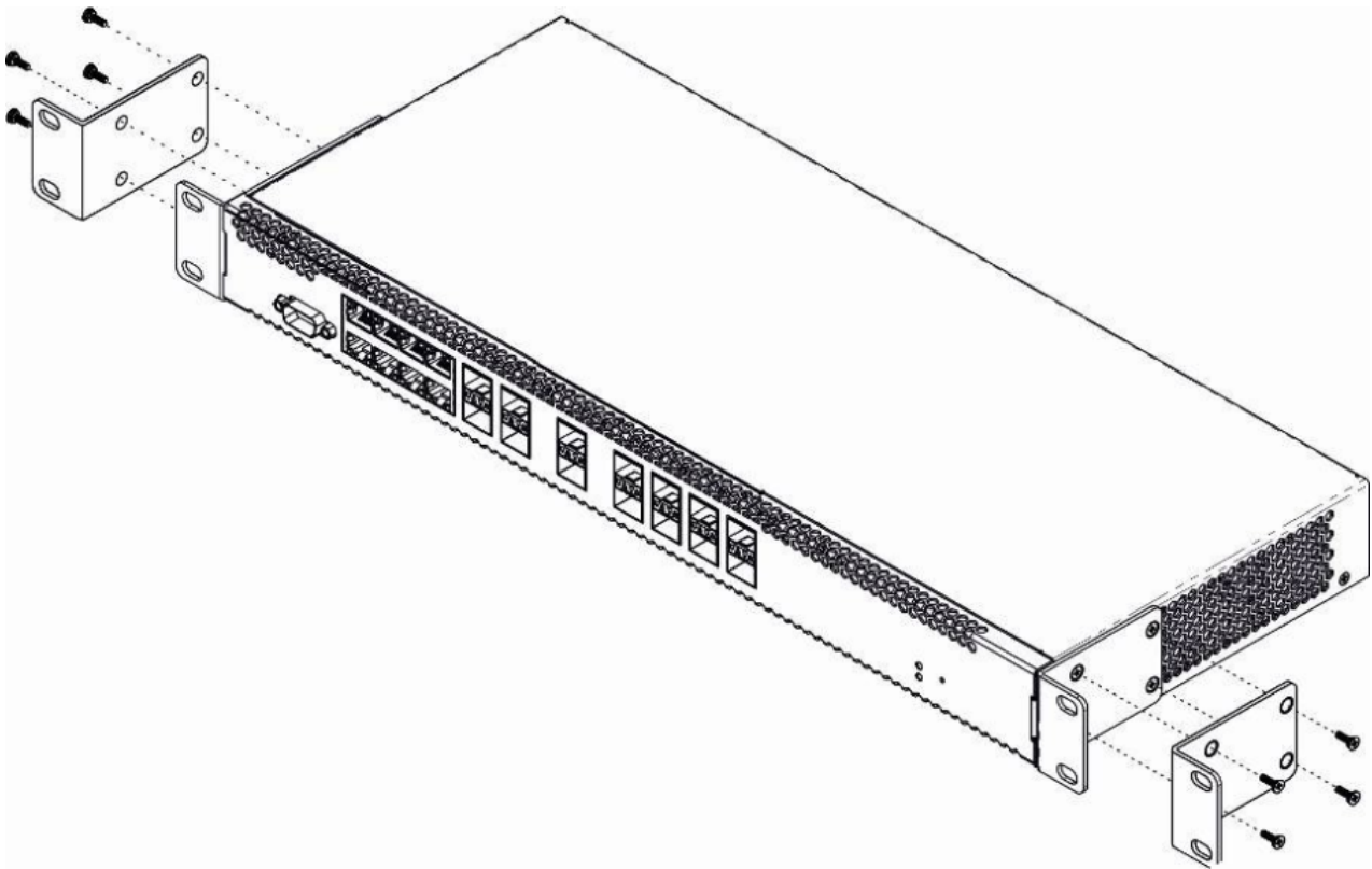
Рисунок 2 — Крепление кронштейнов
