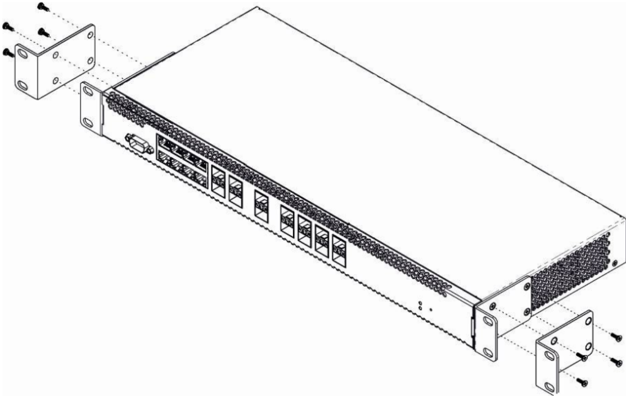
Рисунок 2 — Крепление кронштейнов
