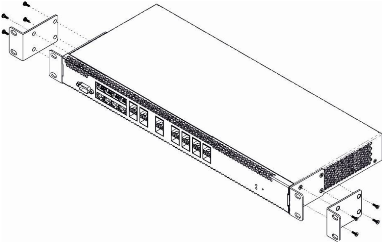
Рисунок 2 — Крепление кронштейнов
