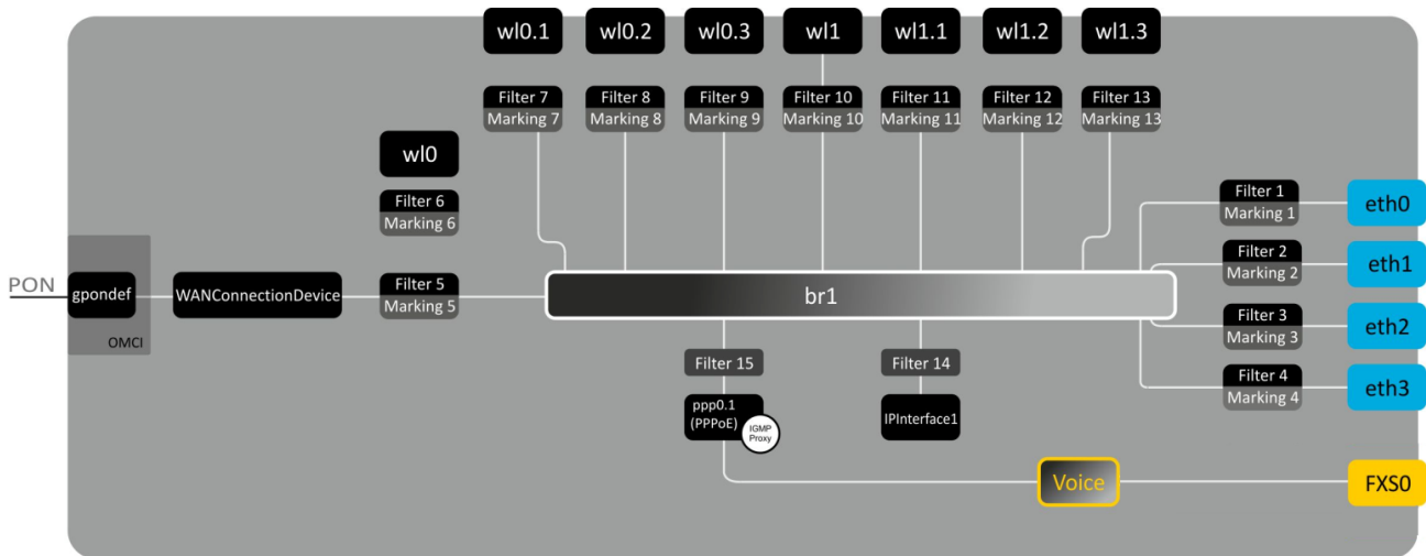
Рисунок 7 – Логическая архитектура устройства с заводской конфигурацией
