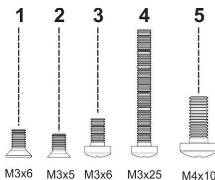
Рисунок 17 – Типы болтов для сборки SMG
