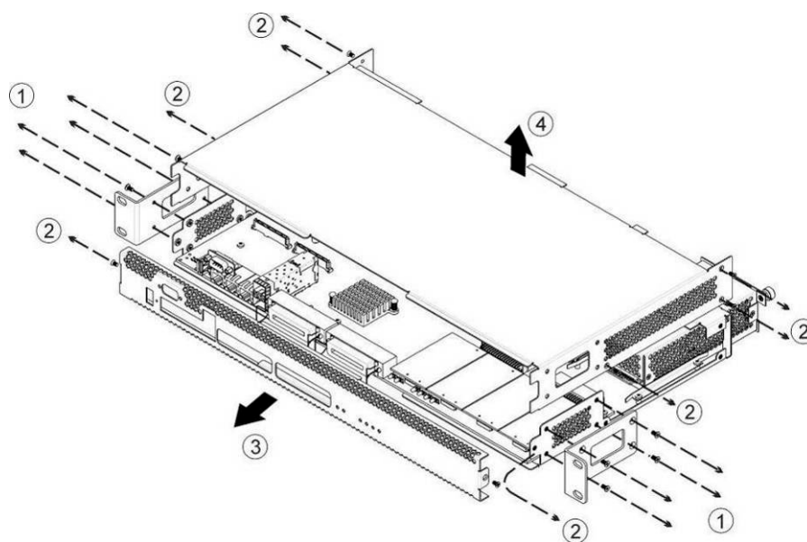
Рисунок 15 – Порядок вскрытия корпуса SMG-1016M
