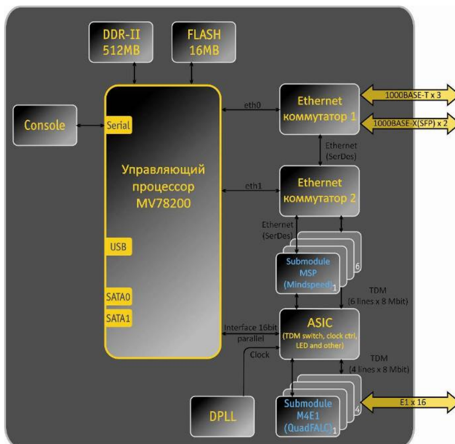
Рисунок 5 – Функциональная схема SMG-1016M
