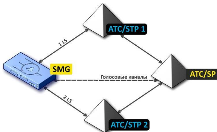
Рисунок 34 – Схема подключения SMG в комбинированном режиме
