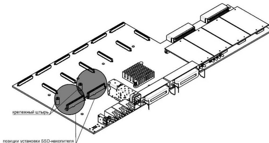
Рисунок 24 – Установка SSD-накопителя
