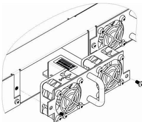
Рисунок 21 – Блок вентиляции SMG-1016M. Крепление в корпус
