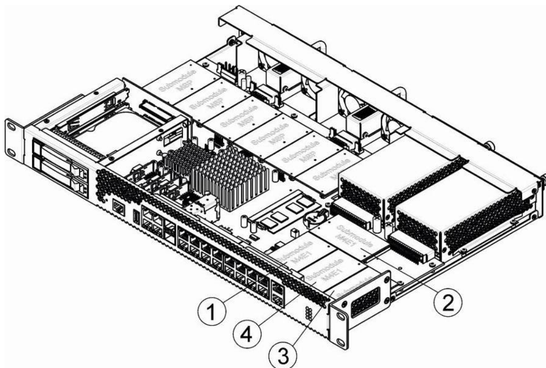
Рисунок 20 – Расположение субмодулей в SMG-2016
