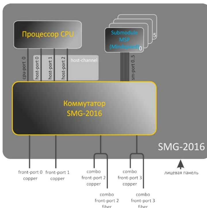
Рисунок 35 – Структура коммутатора
