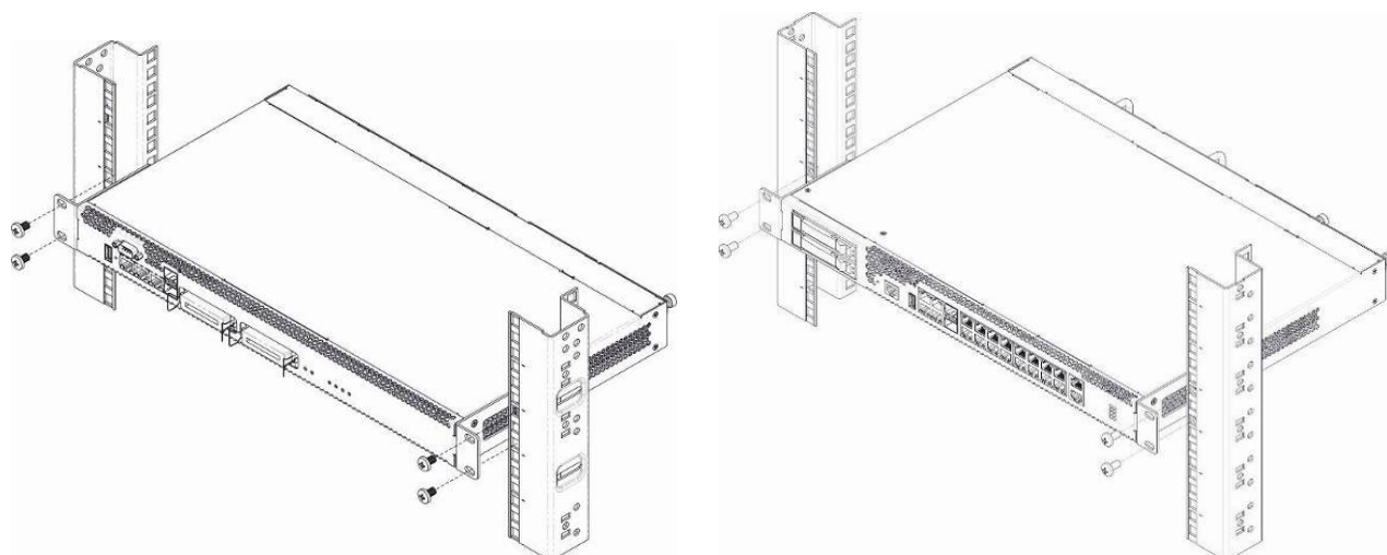
Рисунок 13 – Установка устройства в стойку SMG-1016M(слева) и SMG-2016 (справа)
