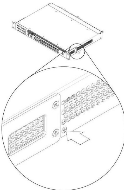
Рисунок 18 – Сборка SMG в корпус
