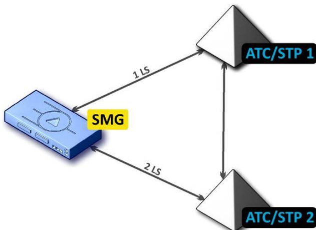
Рисунок 33 – Схема подключения SMG при работе в квазисвязанном режиме через АТС с STP
