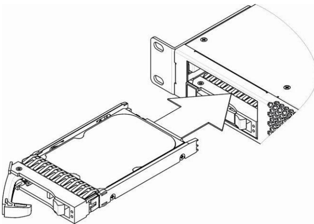
Рисунок 28 – Монтаж SATA-диска в корпус устройства
