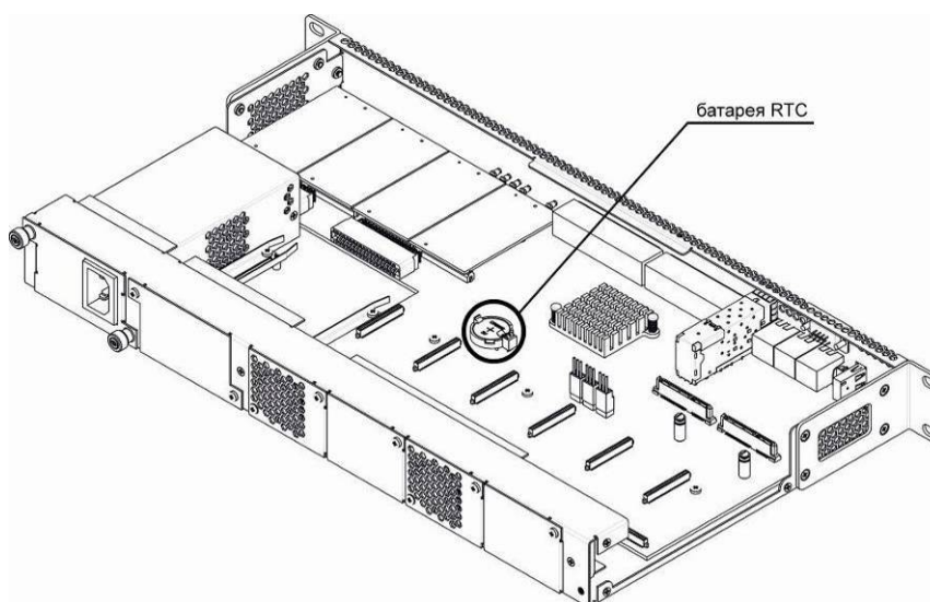
Рисунок 29 – Положение батареи RTC для SMG-1016M
