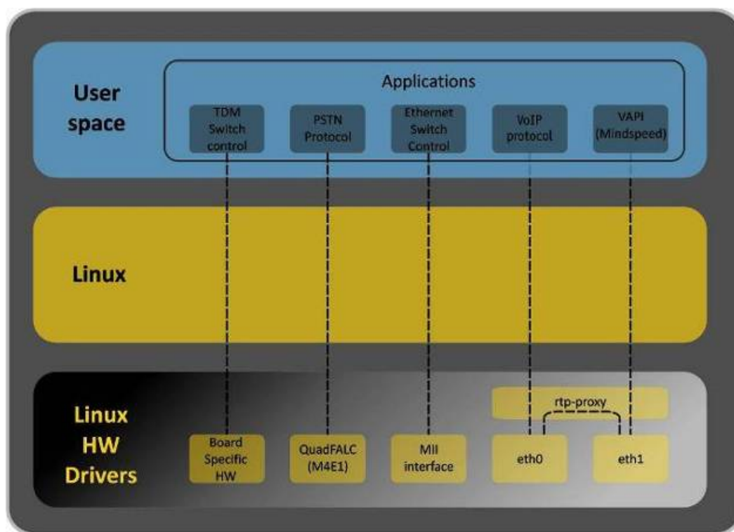
Рисунок 7 – Структура программного обеспечения SMG
