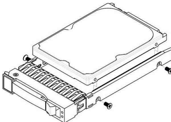
Рисунок 27 – Крепление SATA-диска в лоток направляющих салазок
