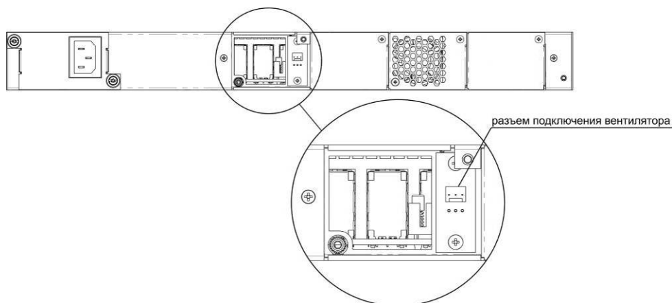
Рисунок 23 – Разъем для подключения вентилятора SMG-1016M
