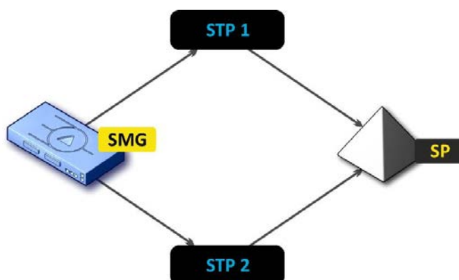
Рисунок 32 – Схема подключения SMG при работе в квазисвязанном режиме через STP
