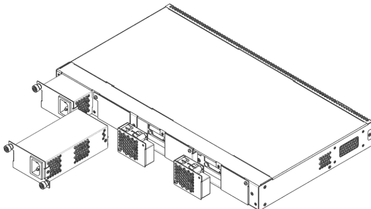
Рисунок 21 – Блок вентиляции SMG-1016M. Крепление в корпус
