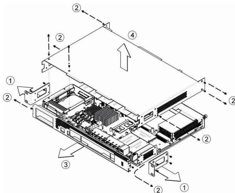
Рисунок 16 – Порядок вскрытия корпуса SMG-2016
