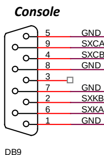
Рисунок 37 – Назначение контактов разъема Console
