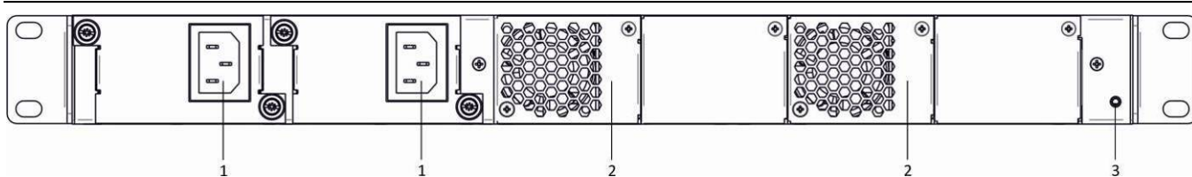
Рисунок 9 – Внешний вид задней панели SMG-1016M
