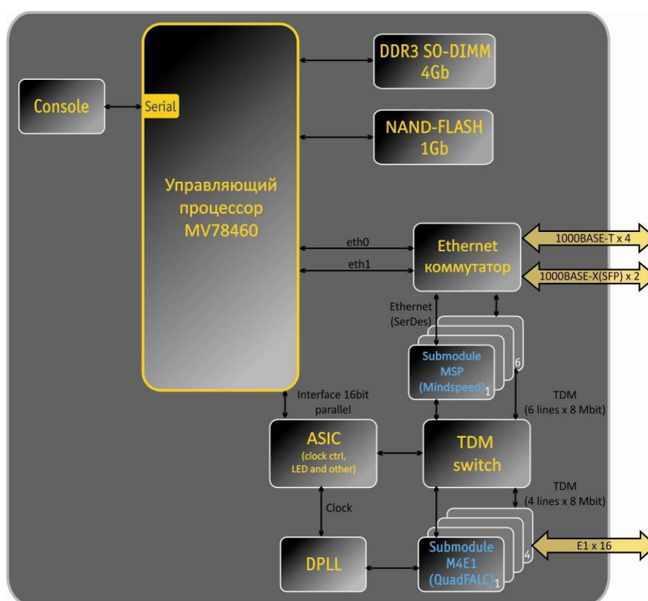
Рисунок 6 – Функциональная схема SMG-2016
