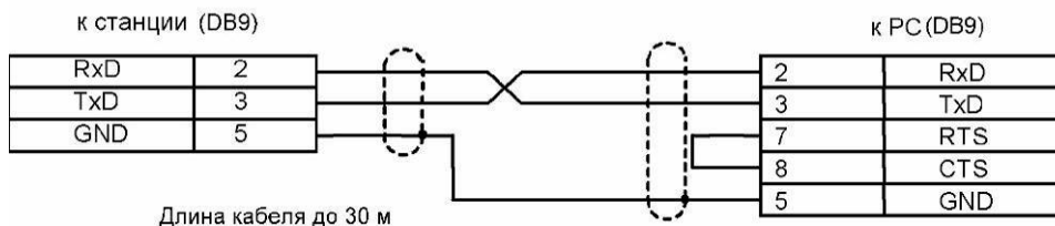
Рисунок 38 – Схема кабеля для подключения к ПОРТ1, ПОРТ2
