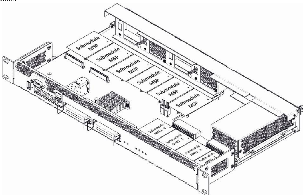
Рисунок 19 – Расположение submodule'ов в SMG-1016M
