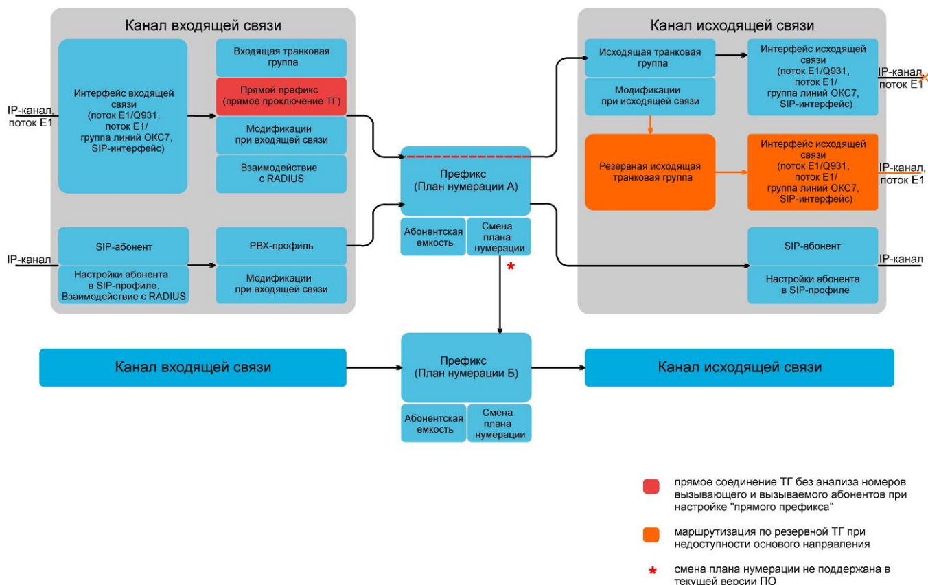
Рисунок 40 – Взаимосвязь параметров маршрутизации, абонентов и СЛ
