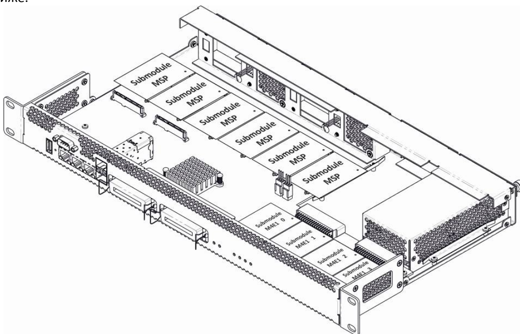
Рисунок 19 – Расположение субмодулей в SMG-1016M
