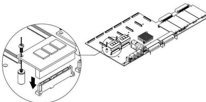
Рисунок 25 – Монтаж SSD-накопителя
