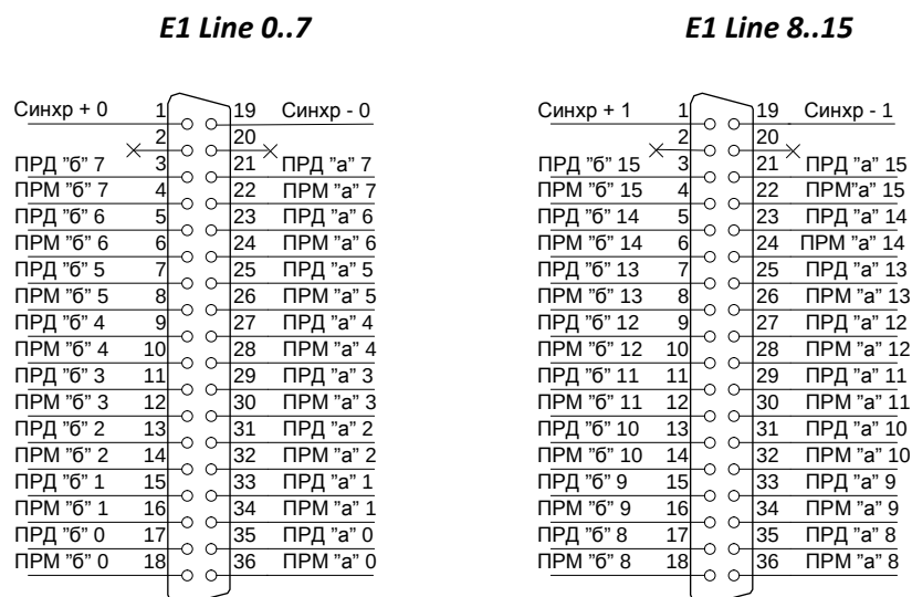
Рисунок 36 – Назначение контактов разъемов E1 Line
