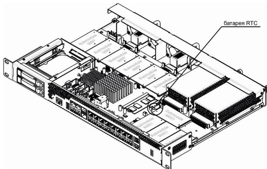
Рисунок 30 – Положение батареи RTC для SMG-2016
