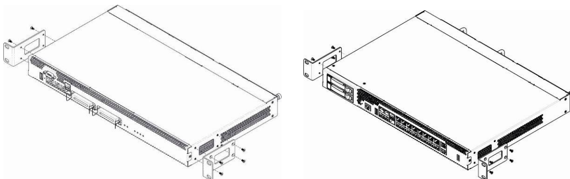
Рисунок 12– Крепление кронштейнов для SMG-1016M(слева) и SMG-2016 (справа)
