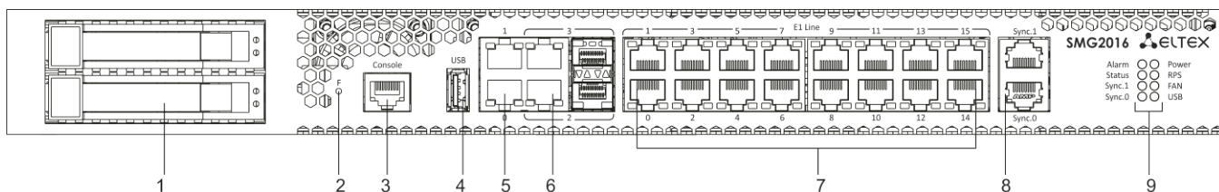
Рисунок 10 – Внешний вид передней панели SMG-2016
