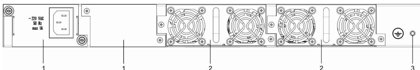
Рисунок 11 – Внешний вид задней панели SMG-2016
