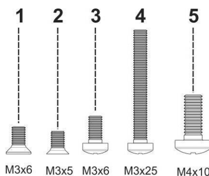
Рисунок 17 – Типы болтов для сборки SMG
